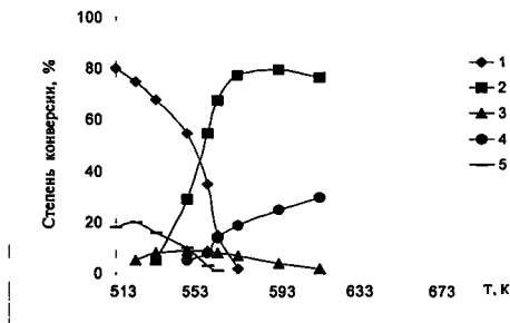
Рис.13. Соотношение продуктов реакции окислительной конверсии этанола на NiNaY:
