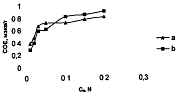
Рис 36 Зависимость COE (Sr 2+ ) и COE (Cs + ) от концентрации растворов для необработанного CL(Ge): а - COE (Cs + ), б - COE (Sr 2+ )
