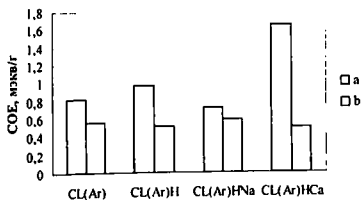
Рис. 42. Диаграмма сравнительных значений COE(Sr^{2+}) для ионообменной сорбции из а) индивидуальных растворов Sr(NO_3)_2 и б) смеси Sr(NO_3)_2 и CsNO_3
