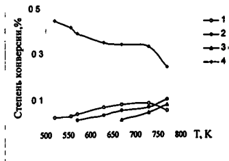
Рис. 58. Соотношение продуктов конверсии метанола на Bi2212: 1 – \text{CH}_2\text{O} ; 2 – \text{CO} ; 3 – \text{CO}_2 ; 4 – \text{CH}_3\text{OH}
