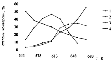
Рис 18 Температурная зависимость выхода продуктов конверсии этанола на AgCl. 1 – C 2 H 5 OH, 2 – CH 3 CHO, 3 – C 2 H 4 , 4 – CO 2
