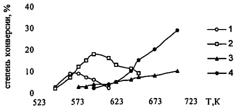
Рис 10. Соотношение продуктов конверсии этанола на исходном NaY цеолите:
