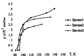
Рис 47 Температурная зависимость удельного сопротивления образцов Y23 приготовленных различными методами 1-№1 (твердофазный метод); 2-№8 (термоллизом из расплава); 3-№9 (метод соосаждения)
