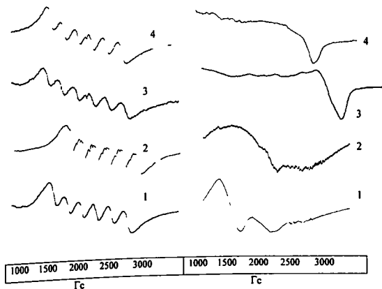
Рис 62 ЭПР-спектр 1- необраб CL(Ge) 2- дегидрат CL(Ge) , 3- CL(Ge)HCu , 4- дегидрат CL(Ge)HCu
