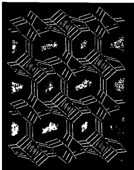
Вид решетки вдоль [001]
