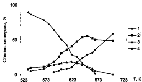
Рис. 19. Окислительное превращение этанола на CuCl : 1 – C_2H_5OH ; 2 – C_2H_4 ; 3 – CH_3CHO ; 4 – CO_2 ;
