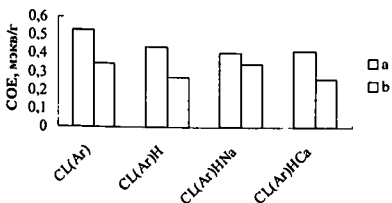
Рис 43 Диаграмма сравнительных значений COE(Cs^+) для ионообменной сорбции из: а) индивидуальных растворов CsNO_3 и б) смеси Sr(NO_3)_2 и CsNO_3
