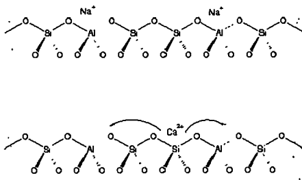
Рис 1. Компенсирующие отрицательный заряд решетки цеолита катионы щелочных и щелочноземельных металлов.
