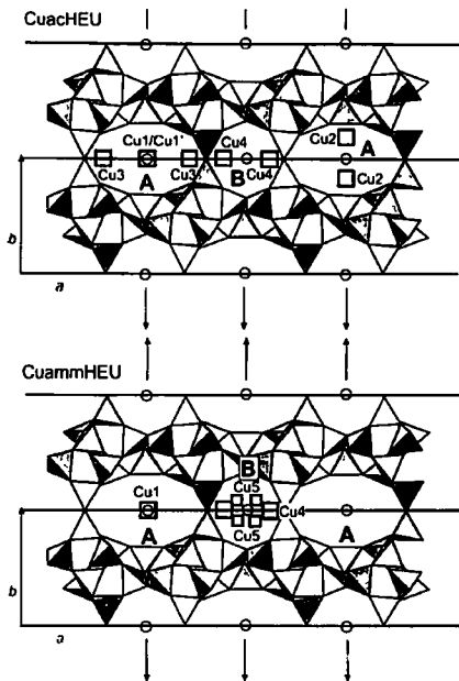
Рис 6. Полиэдрическая модель, отображающая фрагмент структуры CL (HEU) с внекристаллическими ионами \text{Cu}^{2+}
