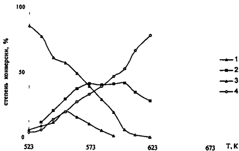
Рис. 19. Окислительное превращение этанола на CuCl : 1 – C_2H_5OH ; 2 – C_2H_4 ; 3 – CH_3CHO ; 4 – CO_2 ;
