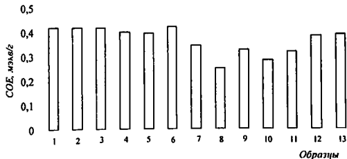
Рис 39. Сорбционная активность изученных образцов в отношении ионов Cs^{2+} : 1-CL(Ar); 2- 10^{12} ; 3 - 10^{13} ; 4- 10^{14} , 5 - 10^{15} , 6 - HCL(Ar), 7 - CaCL(Ar); 8 - NaCL(Ar) \epsilon -облученный, 9 - CaCL(Ar) \epsilon -облученный; 10 - CL(Ar)H + ( \gamma -облученный), 11-14 - Ba CL(Ar)- \epsilon -облученные.
