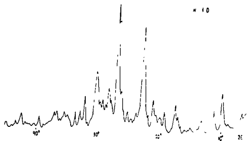
Рентгенограмма исходного необработанного Si (Ar)
