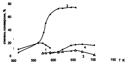
Рис 12. Соотношение продуктов конверсии этанола на \text{CoMnNaY} : 1 – (\text{C}_2\text{H}_5)_2\text{O} ; 2 – \text{C}_2\text{H}_4 ; 3 – \text{CH}_3\text{CHO} ; 4 – \text{CO}_2
