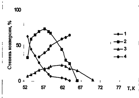
Рис. 21. Температурная зависимость продуктов конверсии этанола на \text{CoCl} : 1 - \text{C}_2\text{H}_5\text{OH} ; 2 - \text{C}_2\text{H}_4 ; 3 - \text{CH}_3\text{CHO} , 4 - \text{CO}_2
