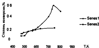
Рис 59. Кривые общей конверсии спирта на 1 – \text{Y123} ; 2 – \text{Bi2212} .
