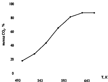
Рис.17. Окислительное превращение этанола до \text{CO}_2 на CuHZSM
