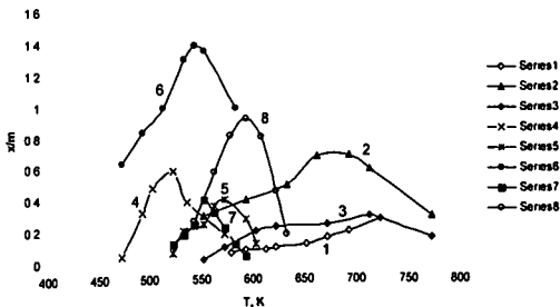
Рис 65 Температурная зависимость удельной активности по ацетальдегиду некоторых из изученных катализаторов: 1 – NaY, 2 – Y123, 3 – Bi2212; 4 – CuNaY, 5 – CoNaY, 6 – AgNaY; 7 – CuCL, 8 – AgCL.
