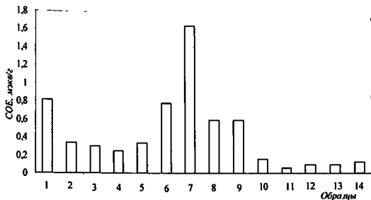
Рис 38. Сорбционная активность изученных образцов в отношении ионов Sr^{2+} : 1-CL(Ar); 2- 10^{12} , 3 - 10^{13} ; 4- 10^{14} , 5 - 10^{15} , 6 - HCL(Ar); 7 - CaCL(Ar); 8 - NaCL(Ar) \epsilon -облученный, 9 - CaCL(Ar) \epsilon -облученный, 10 - CL(Ar)H + ( \gamma -облученный); 11-14 - Ba CL(Ar)- \epsilon -облученные
