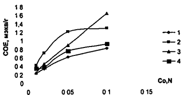
Рис 35. Зависимость COE (Sr 2+ ) от концентрации раствора при соотношении цеолит:раствор 1/100 модифицированных образцов CL(Ar): 1-CL(Ar), 2-CL(Ar)HNa, 3 - CL(Ar)HCa, 4-CL(Ar)H
