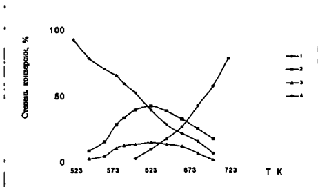
Рис. 22. Температурная зависимость соотношения продуктов конверсии этанола на исходном \text{CL} : 1 - \text{C}_2\text{H}_5\text{OH} ; 2 - \text{C}_2\text{H}_4 ; 3 - \text{CH}_3\text{CHO} ; 4 - \text{CO}_2
