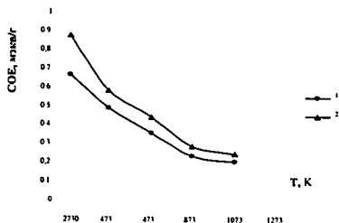
Рис. 34 Зависимость COE(Sr^{2+}) от температуры термообработки образцов (концентрация рабочих растворов 0.01N при соотношении цеолит.раствор 1:100) CL (Ar), 2 – CL(Ge)
