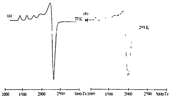
Рис.62 ЭПР-спектры гидратированных образцов CL(Ge)НСu, снятых при 293 и 77 К.
