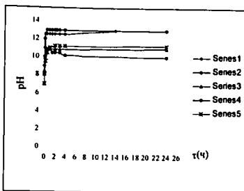
Рис 54. Зависимость pH смеси от времени выдержки порошков ВТСП и температуры: 1 – Y 123(298 K), 2 – Y 123(353 K), 3 – Bi 2122(298 K); 4 – Bi 2122(353 K), 5 – Y 123(обр. №2 таблетир ).
