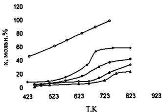
Рис 23. Температурная зависимость степени конверсии \text{NO}_x на модифицированном CL ○ - CuCL; ◆ - CL; ● - NiCL; ◇ - CoCL, ▲ - HCL
