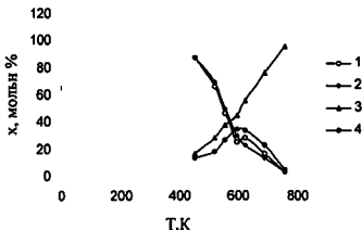
Рис. 27. Соотношение продуктов реакции (\text{NO}+\text{NO}_2)+\text{H}_2 : 1 - \text{NO}+\text{NO}_2 ; 2 - \text{H}_2 ; 3 - \text{N}_2 ; 4 - \text{N}_2\text{O} .
