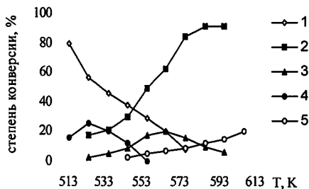
Рис.11. Соотношение продуктов конверсии этанола на \text{CoNaY} 1 – \text{C}_2\text{H}_5\text{OH} , 2 – \text{C}_2\text{H}_4 , 3 – \text{CH}_3\text{CHO} ; 4 – (\text{C}_2\text{H}_5)_2\text{O} ; 5 – \text{CO}_2
