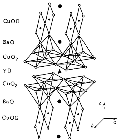
Рис 7 Кристаллическая структура \text{YBa}_2\text{Cu}_3\text{O}_{6.5+\delta} \delta \approx 0.5 ● — Ba ▲ — Y, · — Cu, ○ — O
