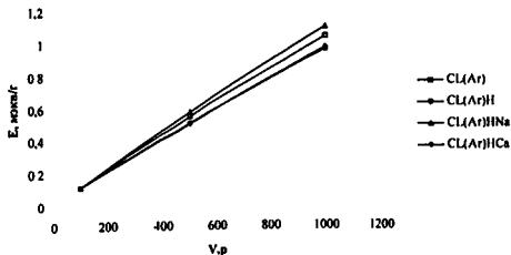
Рис 41. Зависимость COE(Cs^+) от объема смеси растворов раствора По стронцию величина сорбции возрастает постоянно с увеличением соотношения цеолит: раствор
