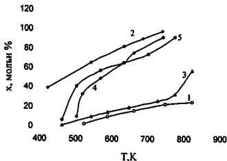
Рис. 26 Температурная зависимость степени разложения \text{NO}_x (O - 1), и в совместной конверсии с CO (◆ - 2), \text{CH}_4 (▲ - 3), \text{H}_2 (◇ - 4) и \text{NH}_3 (● - 5) на CuCl
