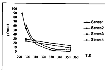
Рис 55 Зависимость времени полного гидролиза от температуры ◦ – теоретическая кривая; • – Y 123 (порошок); ◊ – Bi 2122 (порошок), ◆ I – Y 123 (табл.)
