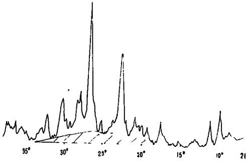
Рентгенограмма CI (Ag)II-600
